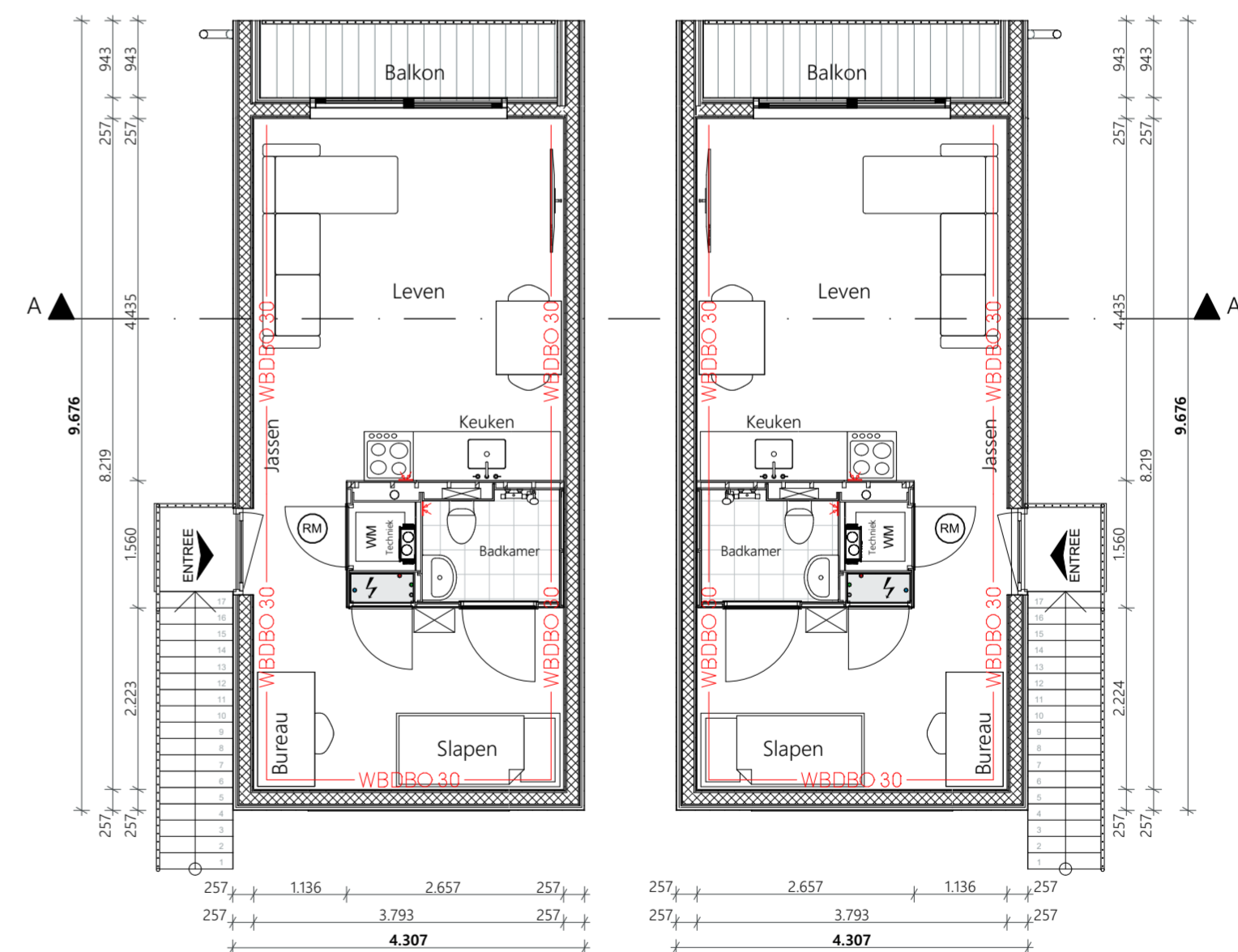
1E VERDIEPING
