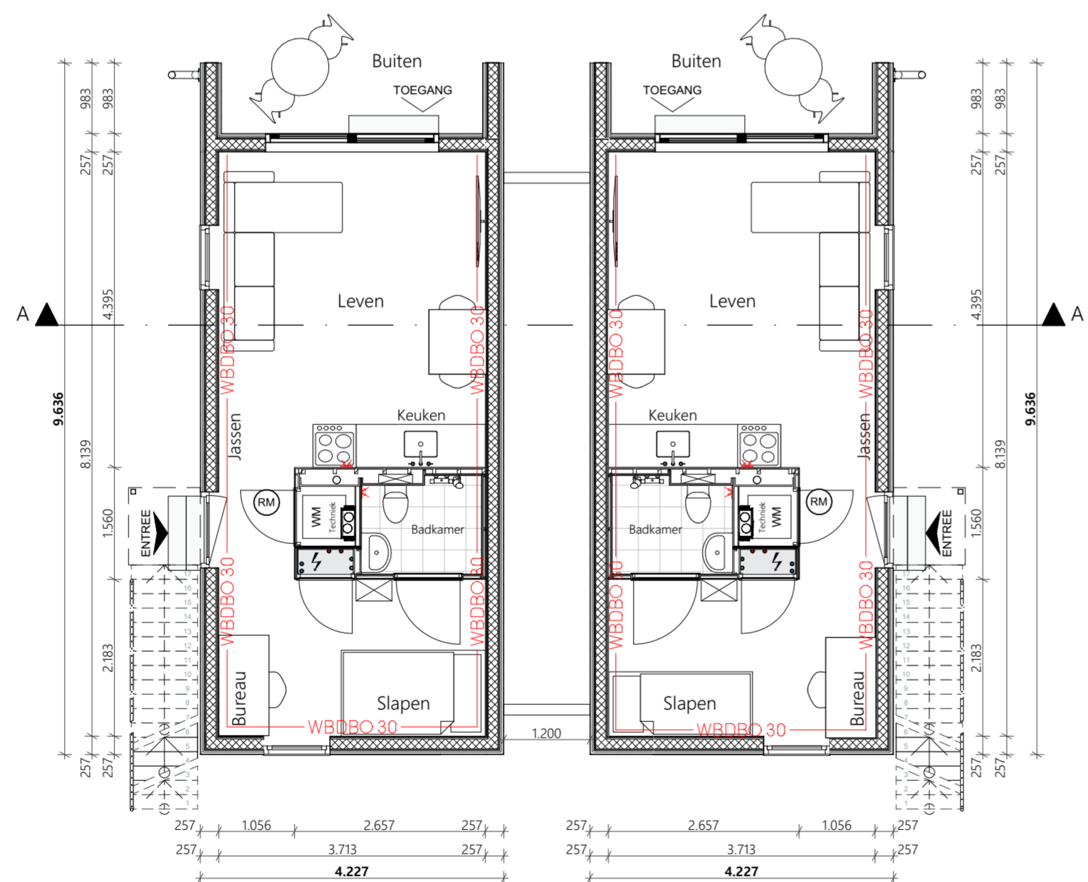
BEGANE GROND
