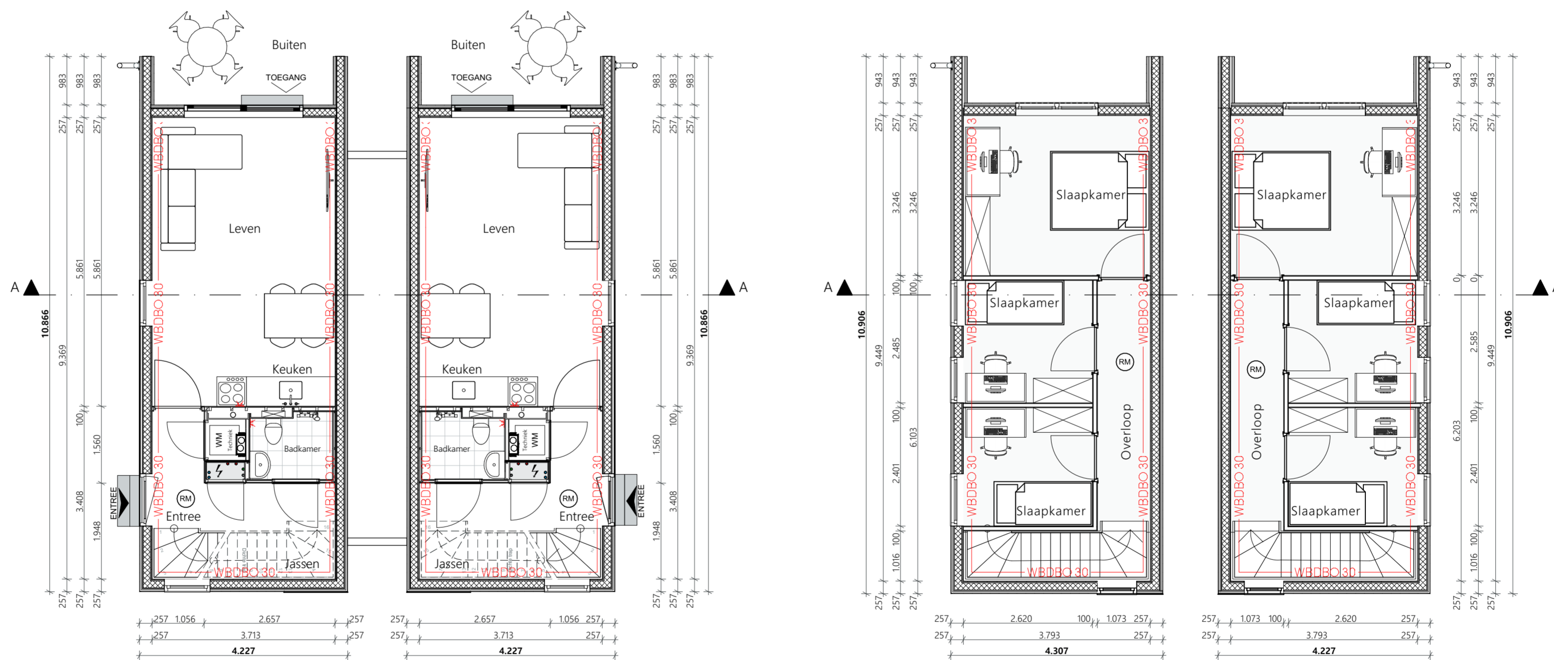
BEGANE GROND
