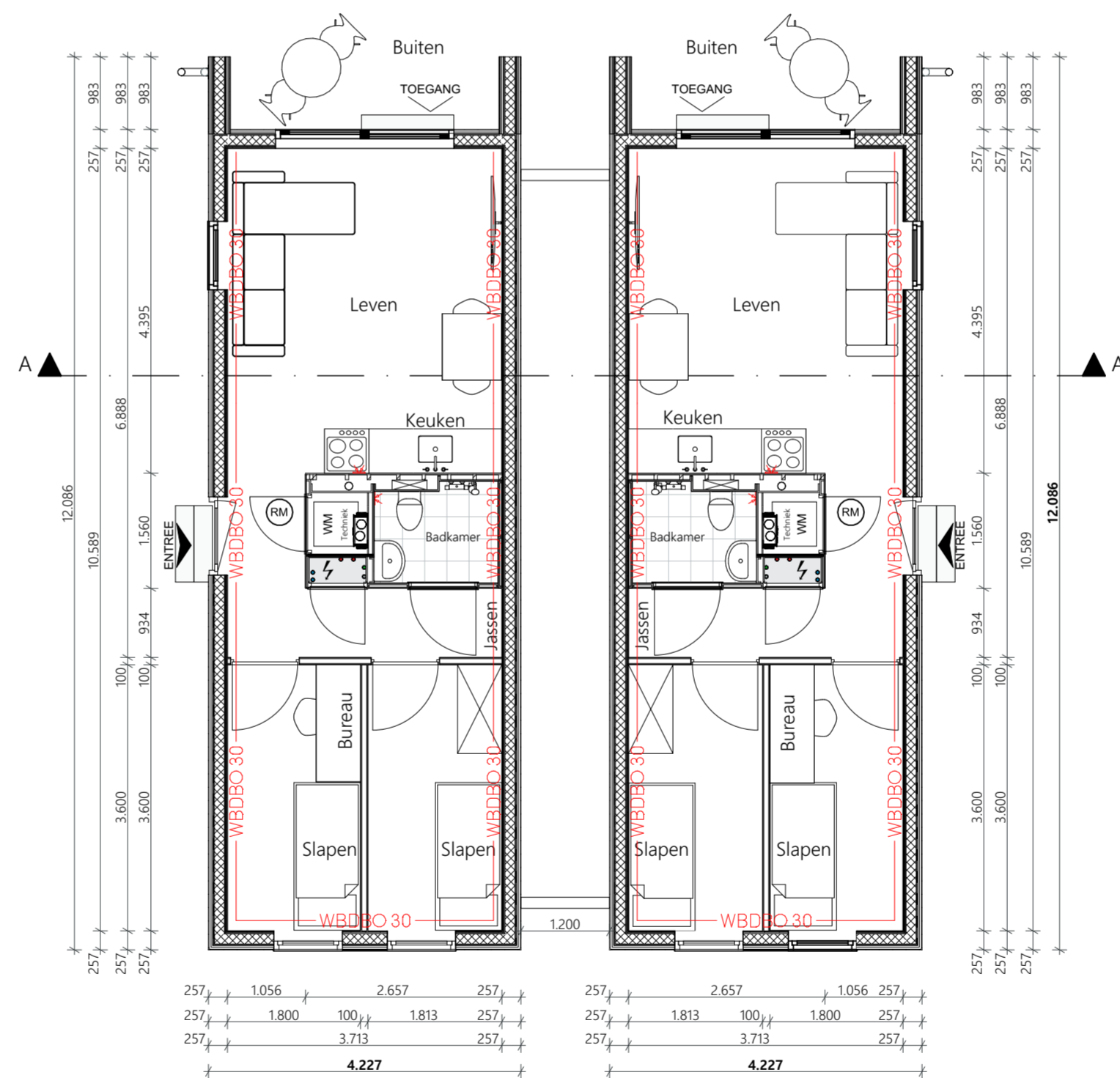
BEGANE GROND
