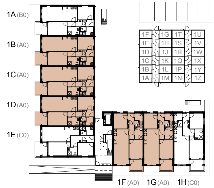
begane grond
