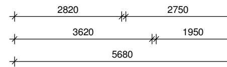
eerste verdieping
