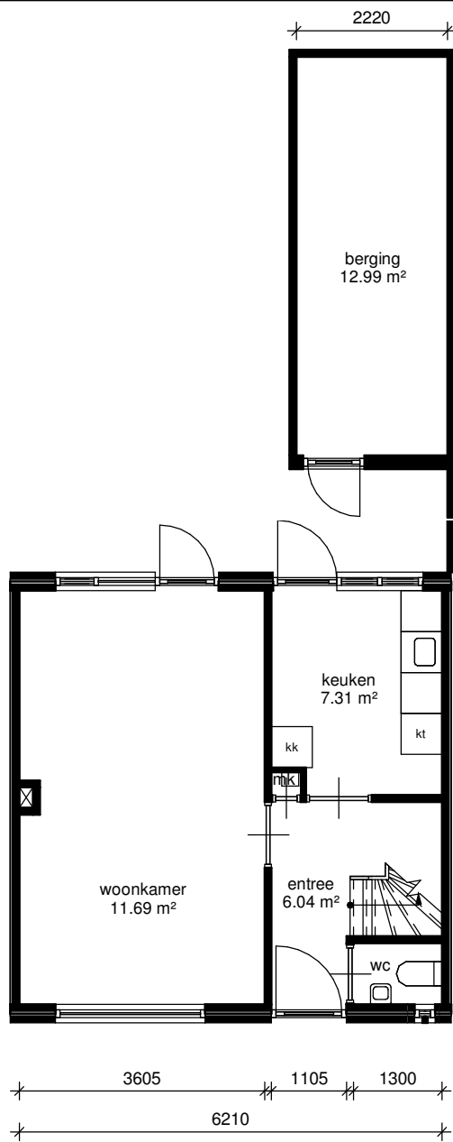
begane grond
